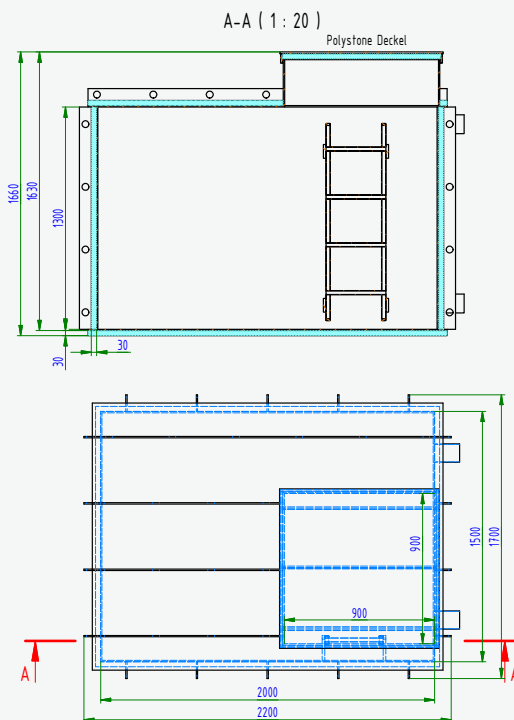
Technikschaft Standard mit Kunststoffdeckel 2,0 x 1,5 x 1,3 m
