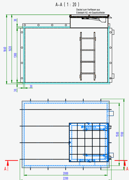
Technikschaft Standard mit Gasdruckfederdeckel 2,0 x 1,5 x 1,3 m
